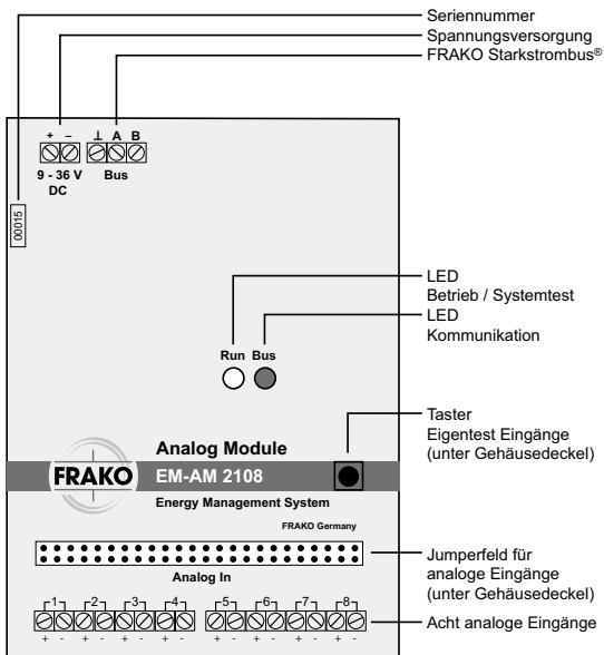
Vorderansicht
