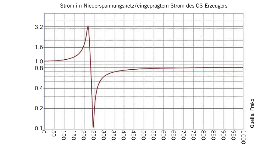
Bild 2: Saugwirkung eines passiven Filtersystems (fr=245 Hz)
