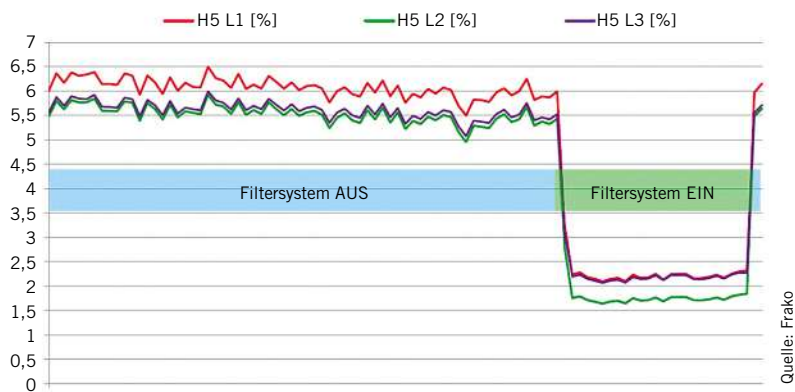
Bild 4: Spannung der 5. Oberschwingung mit und ohne passivem Filtersystem
