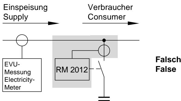
Abb.: Anschluss von Mess- und Hilfsspannung und des Stromwandlers.
