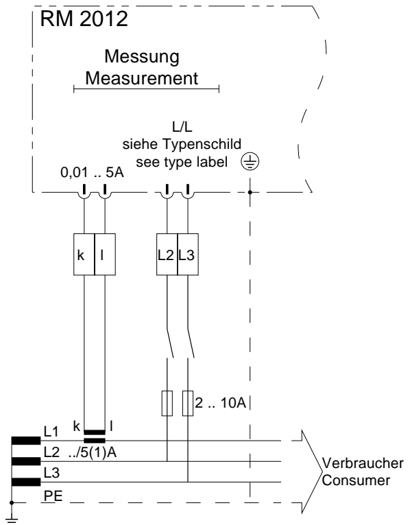
Abb.: Anschluss von Mess- und Hilfsspannung und des Stromwandlers.
