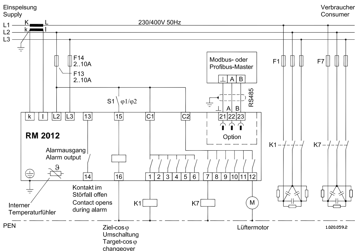
Abb.: Anschlussbeispiel, Blindleistungsregler mit 12 Relaisausgängen, Ziel-cos(phi) Umschaltung und Alarmausgang.
